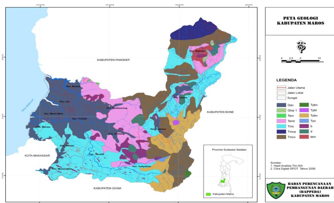
Gambar 2.3 Peta Geologi Kabupaten Maros
