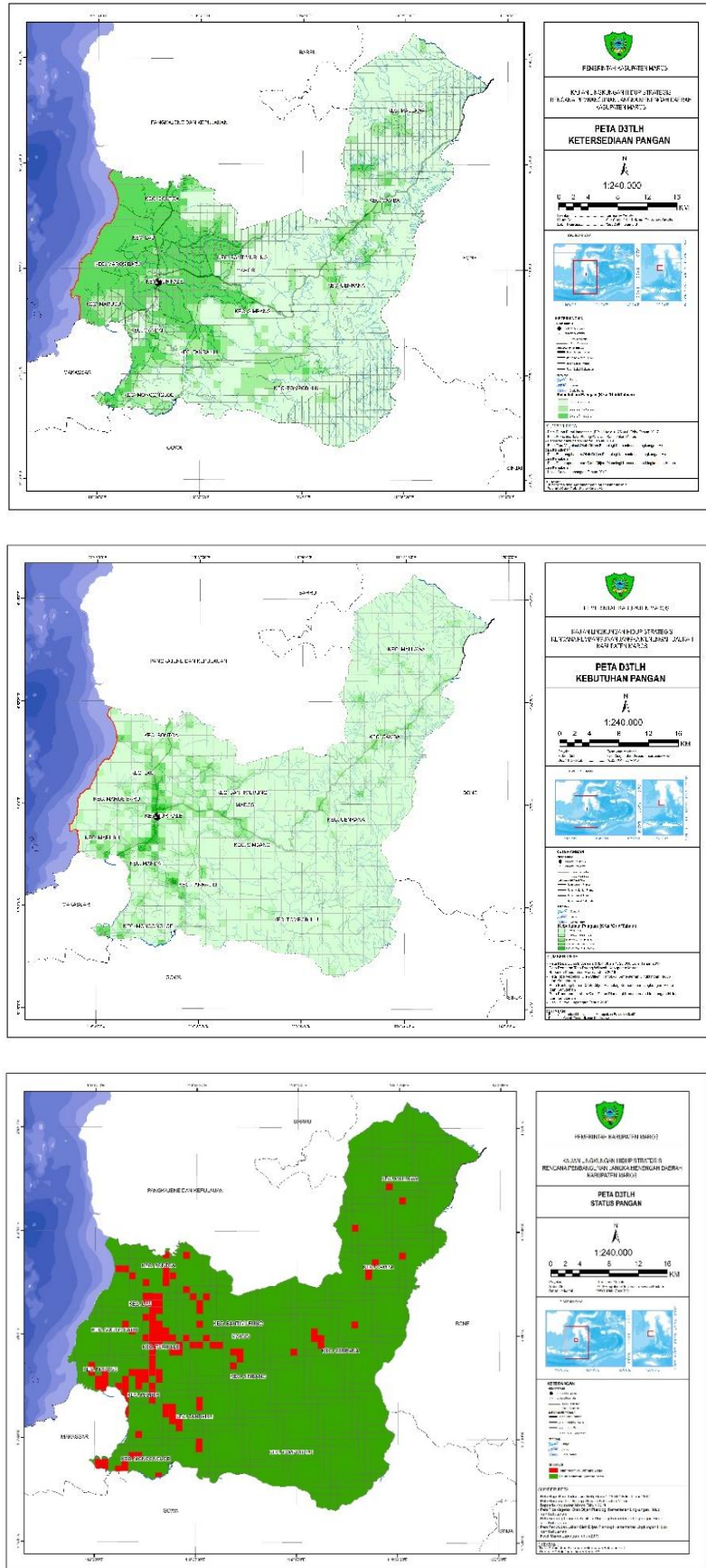
Gambar 2.7 Peta Kajian Daya Dukung Penyediaan Pangan di Kabupaten Maros
