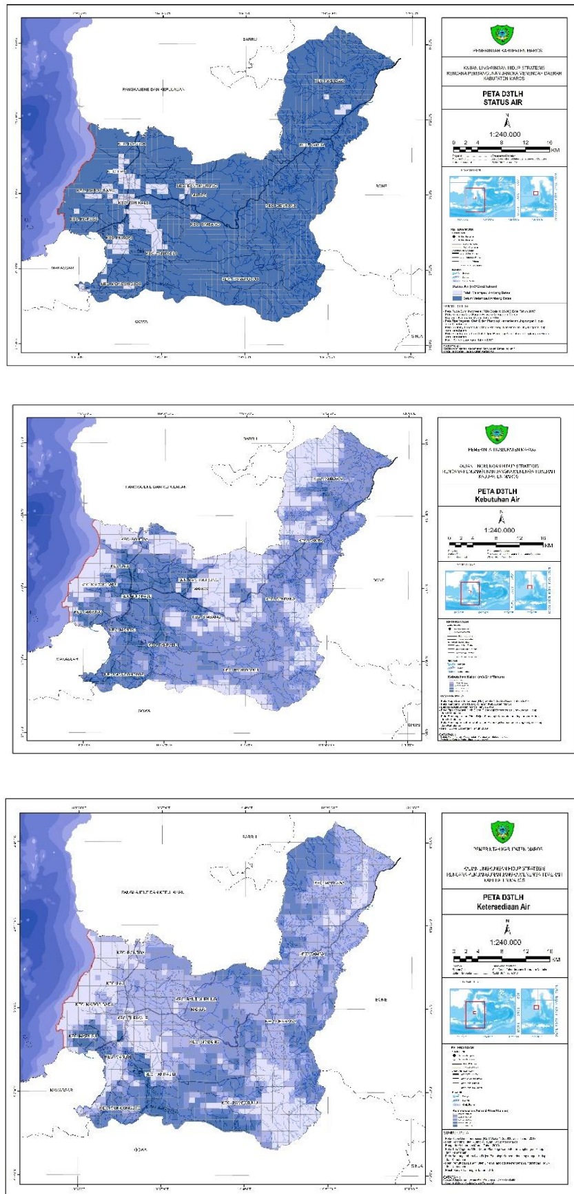
Gambar 2.6 Peta Kajian Daya Dukung Penyediaan Air di Kabupaten Maros
