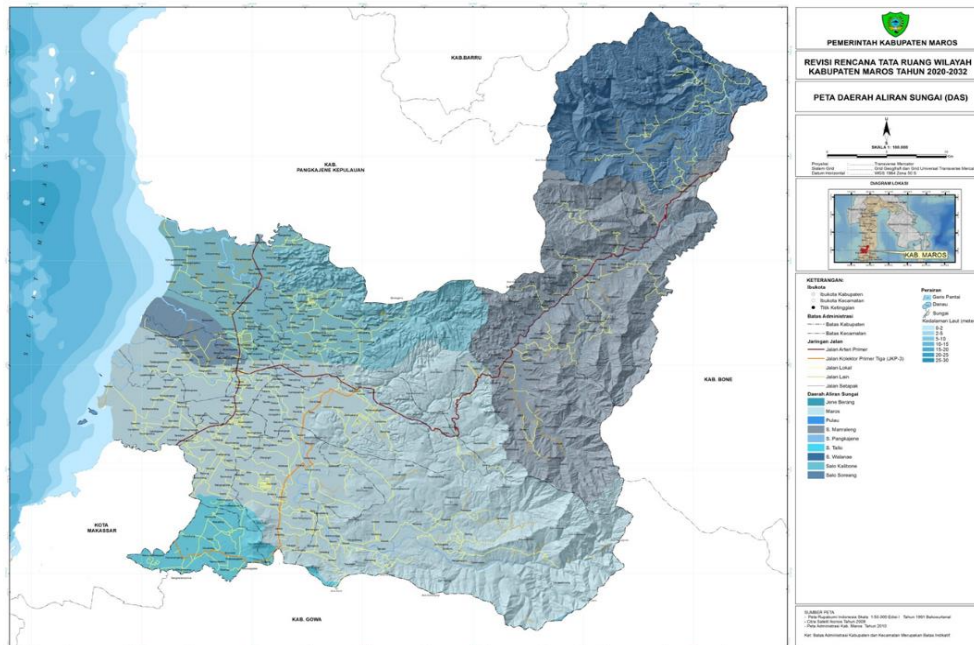
Gambar 2.4 Peta Daerah Aliran Sungai Kabupaten Maros
