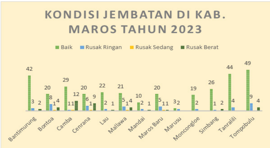
Gambar 49. Diagram Jum- lah dan Kondisi Jembatan di Kab. Maros Menurut Keca- matan Tahun 2023
